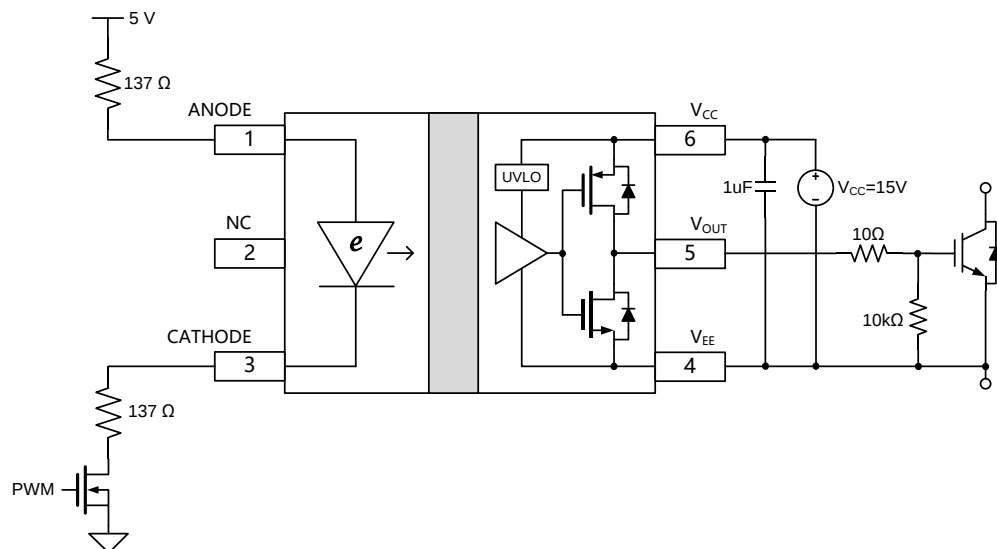
图 9.3 使用单一 MOSFET 作为 CED8262B/CED8262BT 的输入
