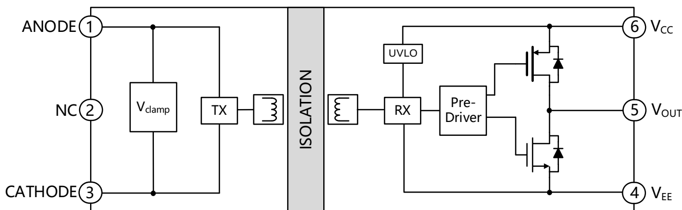
图 9.1 功能框图
