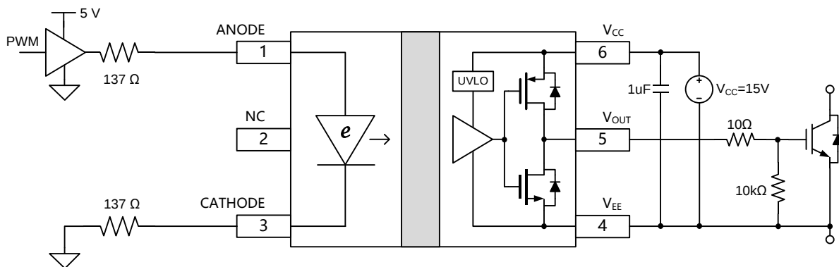
图 9.4 使用 Buffer 电路作为 CED8262B/CED8262BT 的输入
