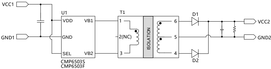
图1. CMP6503S/CMP6503F 单路输出
