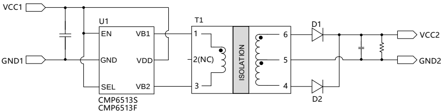
图2. CMP6513S/CMP6513F 单路输出
