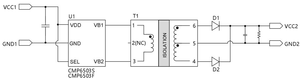
图1. CMP6503S/CMP6503F 单路输出
