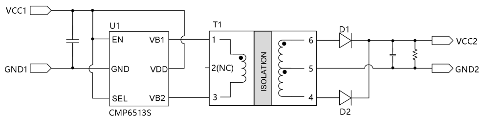
图2. CMP6513S 单路输出
