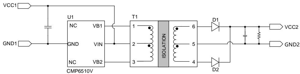
图2. CMP6510V 单路输出
