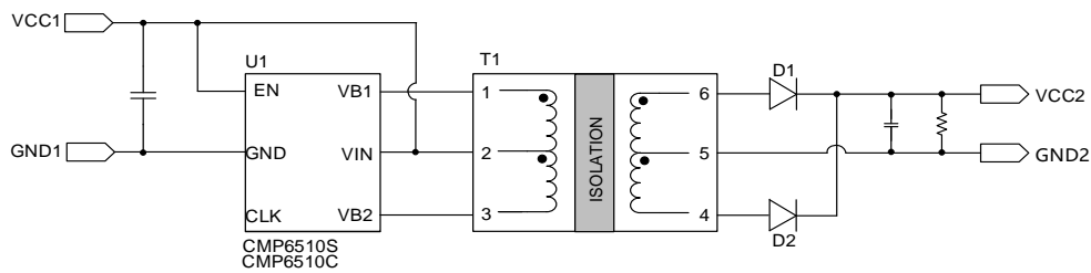
图1. CMP6510S/CMP6510C 单路输出
