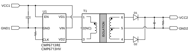
图2.CMP6713RE/CMP6713HV 单路输出
