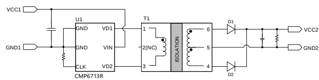
图1. CMP6713R 单路输出
