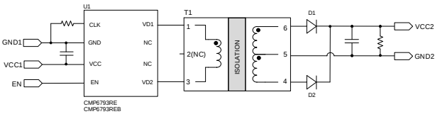
图2. CMP6793RE/CMP6793REB 单路输出
