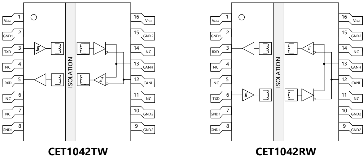
引脚功能
