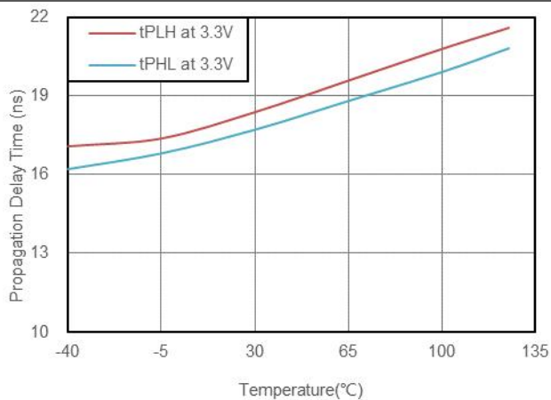
Fig. 8.5. 传输延时 vs. 温度 (3.3V 供电电压)
