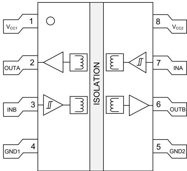
引脚功能
