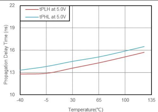
Fig. 8.6. 传输延时 vs. 温度 (5.0V 供电电压)
