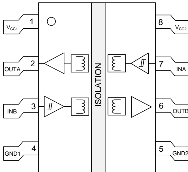
引脚功能
