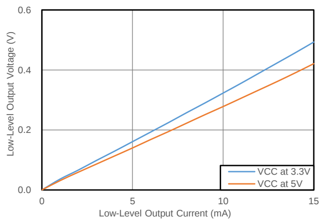
Fig. 8.4. 输出电压 vs. 输出电流
