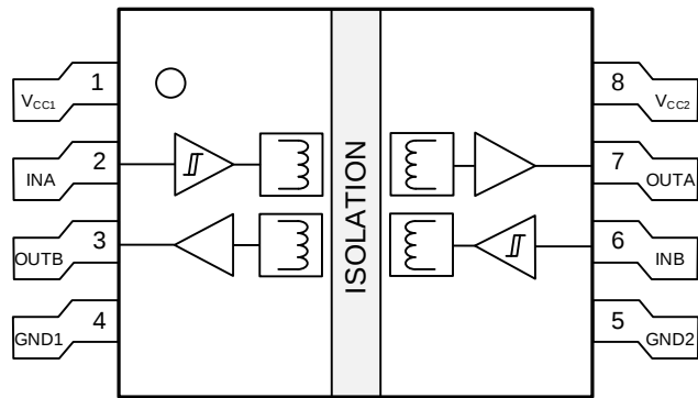
引脚功能
