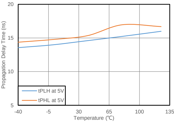
Fig. 8.6. 传输延时 vs. 温度 (5V 供电电压)
