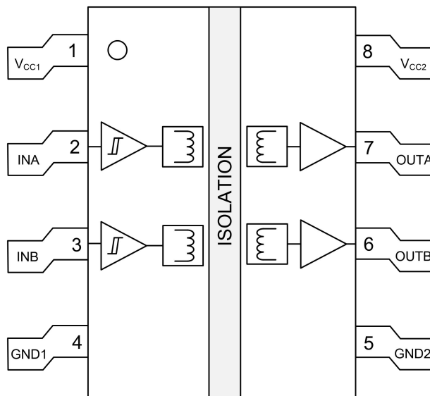
引脚功能
