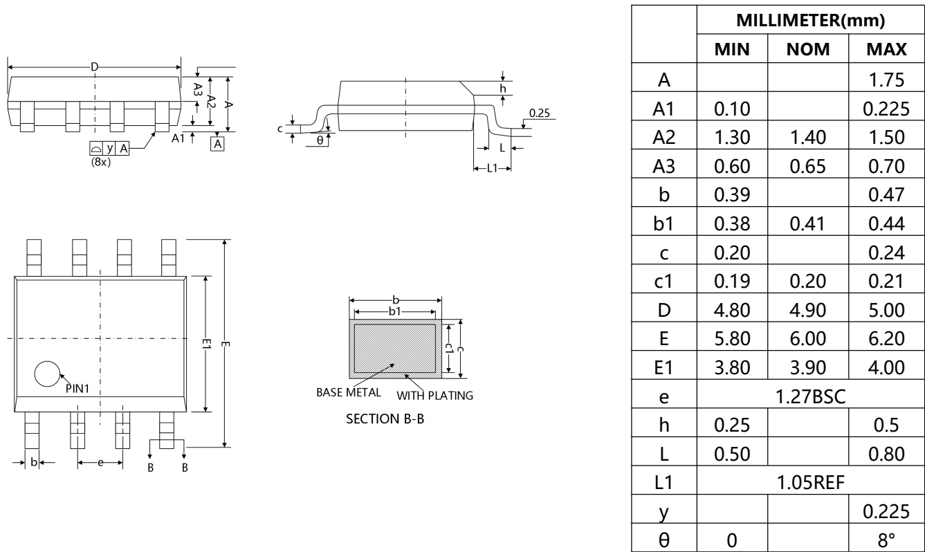
Fig. C1. SOP-8L (150 mil)
