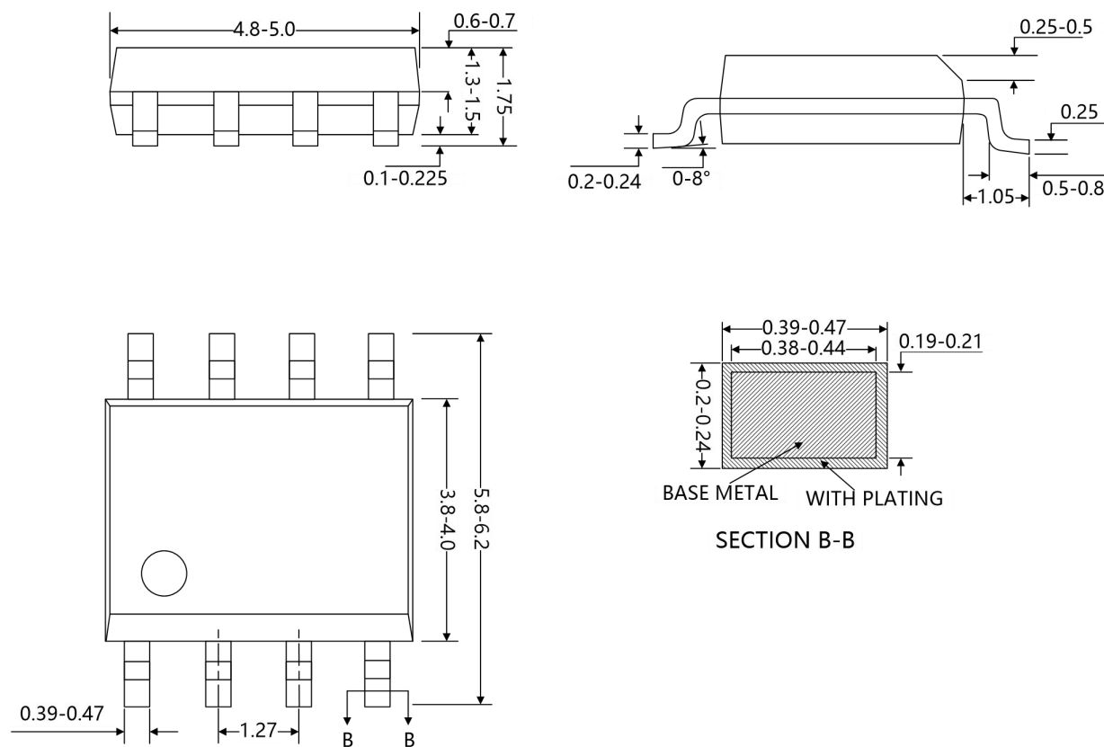
Fig. C1. SOP-8L (150 mil)
