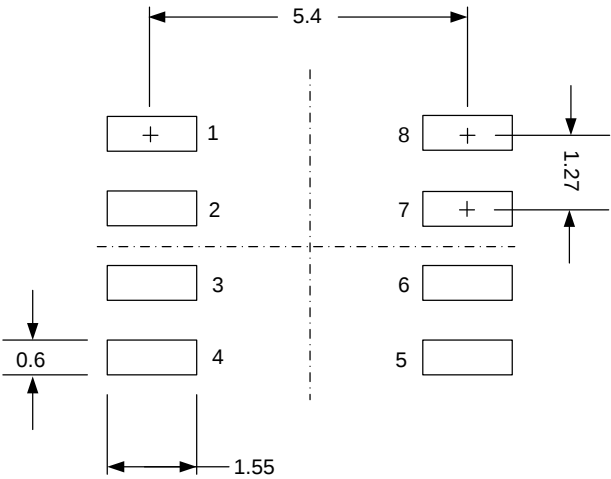
Fig. D1. PCB 焊盘: SOP-8L (150 mil)
