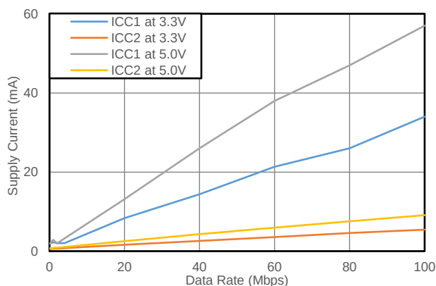
Fig. 8.1. 供电电流 vs. 数据率 (0 pF 负载, 室温)
