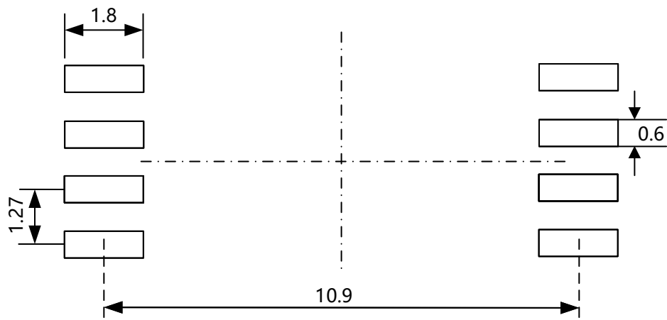
Fig. D1. PCB 焊盘: SOW-8
