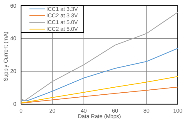
Fig. 8.2. 供电电流 vs. 数据率 (15 pF 负载, 室温)
