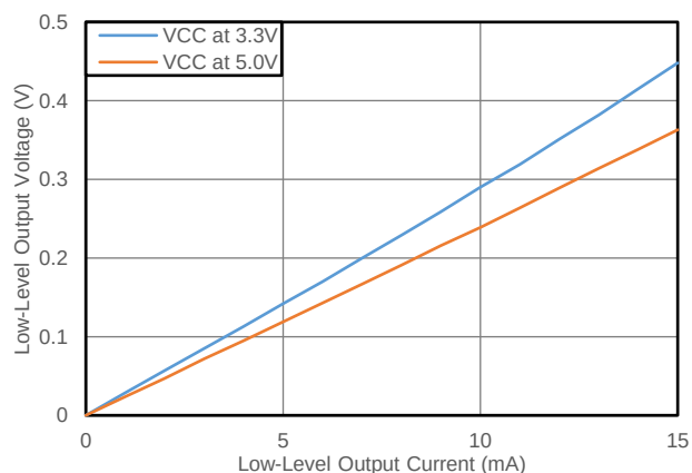
Fig. 8.4. 输出电压 vs. 输出电流
