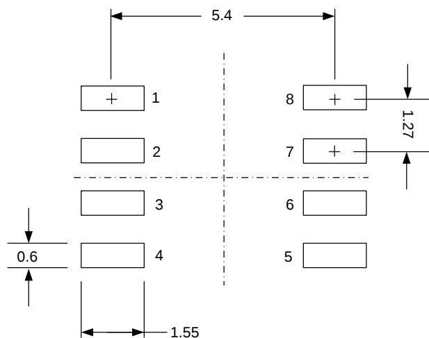
Fig. D1. PCB焊盘: 8-引脚 SOP
