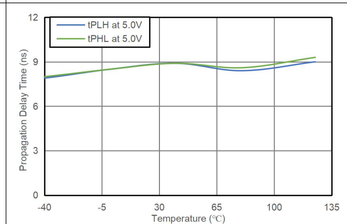
Fig. 8.6. 传输延时 vs. 温度 (5.0V 供电电压)
