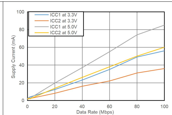
Fig. 8.2. 供电电流 vs. 数据率 (15 pF 负载, 25 °C)
