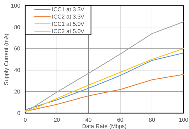
Fig. 8.2. 供电电流 vs. 数据率 (15 pF 负载, 25 °C)
