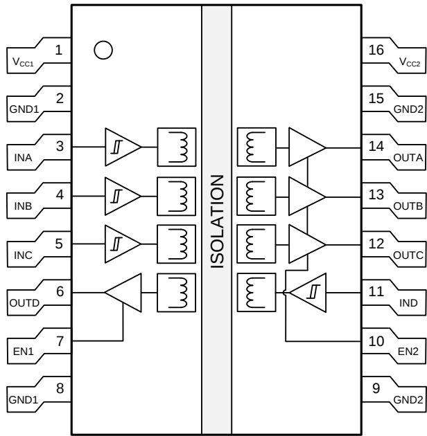
引脚功能
