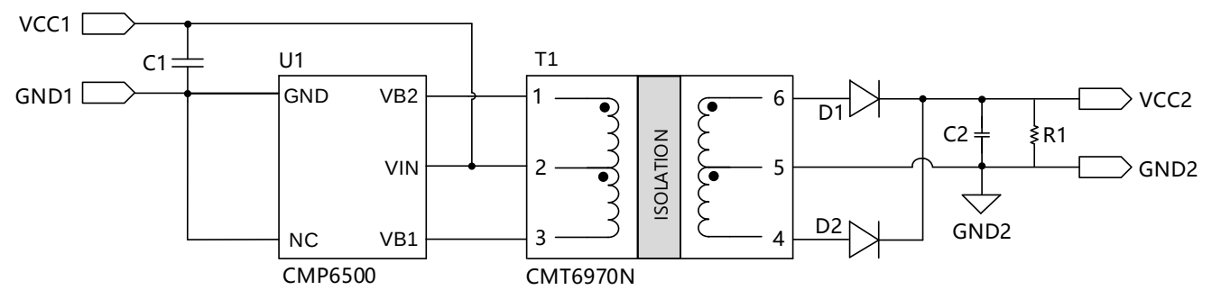
图 8.2 设计原理图
