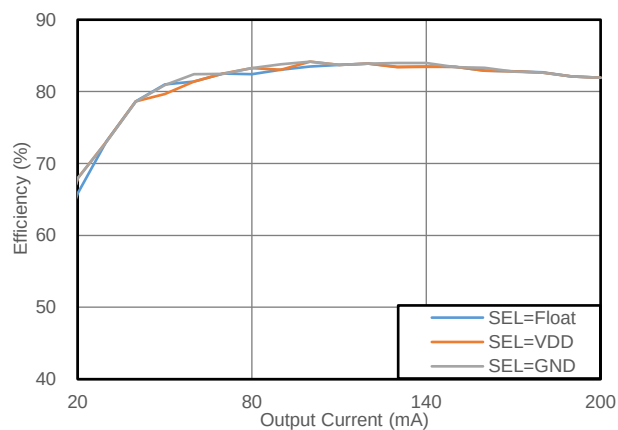
图 8.7 转换效率 vs 输出电流 (CMP6503F+CMT6870N, 5.0V to 5.0V)
