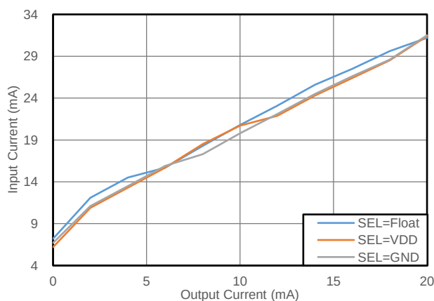
图 8.11 轻载原边供电电流 (CMP6503F+CMT6870N, 5.0V to 5.0V)
