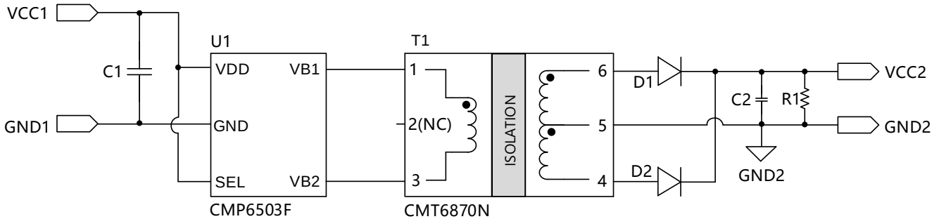
图 7.2 CMP6503F 方案设计原理图
