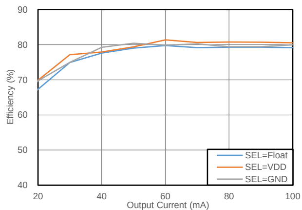
图 8.8 转换效率 vs 输出电流 (CMP6503F+CMT6870N, 3.3V to 3.3V)
