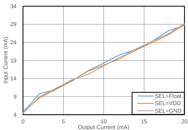
图 8.12 轻载原边供电电流 (CMP6503F+CMT6870N, 3.3V to 3.3V)
