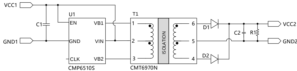
图 8.5 设计原理图
