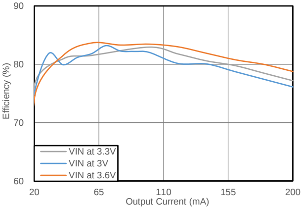
图 7.4 转换效率 vs 输出电流 (常温) (CMP6510S+CMT6970N, 3.3V to 3.3V)
