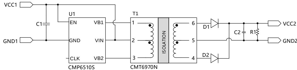
图 8.5 设计原理图
