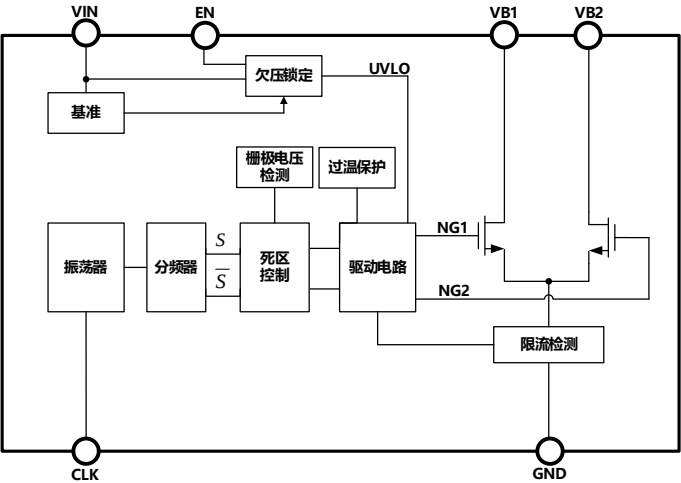
图 8.1 功能框图
