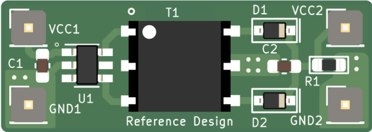
图 8.6 参考 PCB 设计
