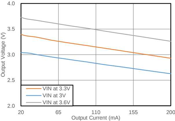
图 7.3 输出电压 vs 输出电流 (常温) (CMP6510S+CMT6970N, 3.3V to 3.3V)
