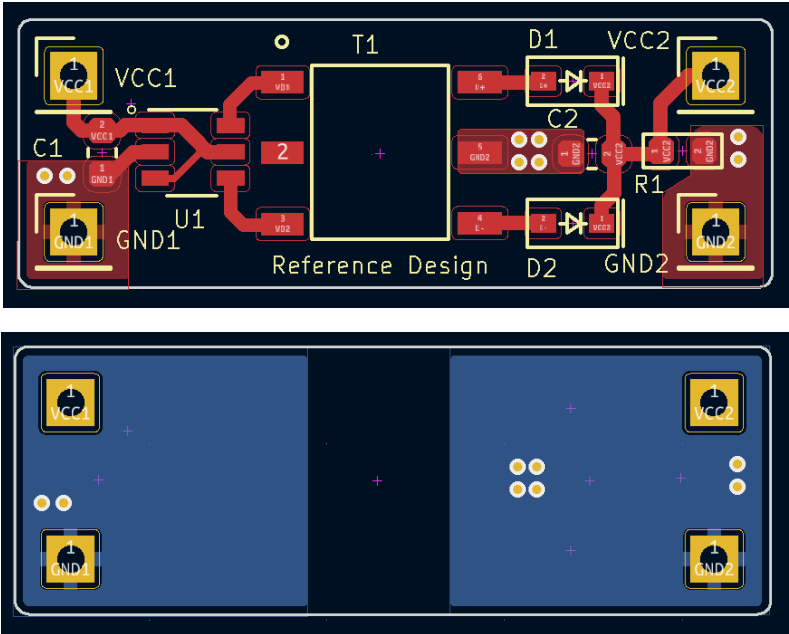
图 8.7 参考 PCB 设计的正反面
