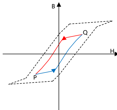
图 8.4 磁芯磁化
