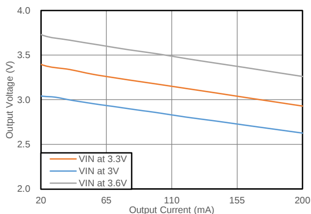
图 7.3 输出电压 vs 输出电流 (室温) (CMP6510V+CMT6970N, 3.3V to 3.3V)
