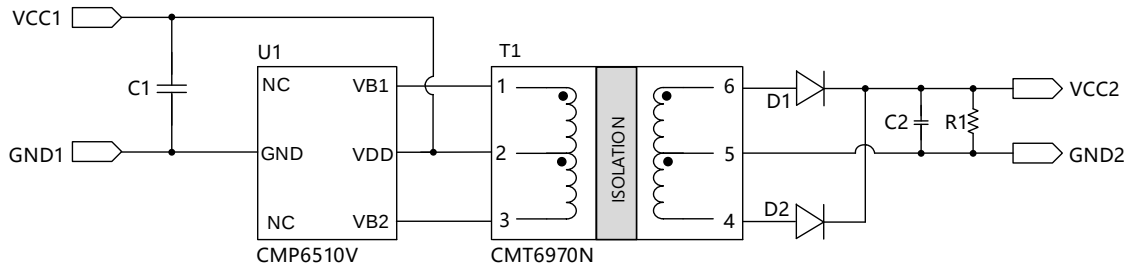
图 8.5 设计原理图
