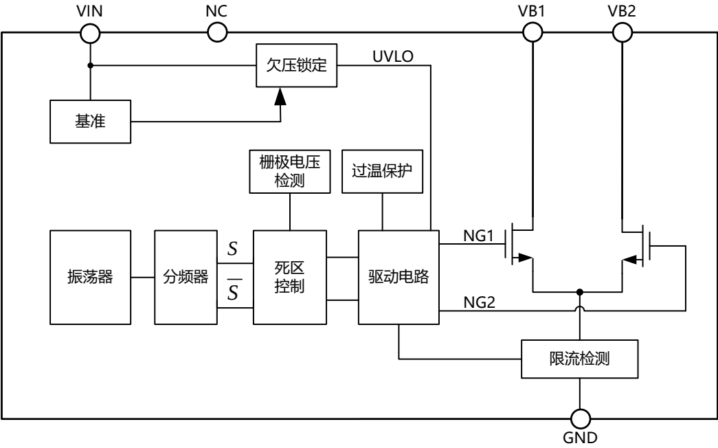
图 8.1 功能框图
