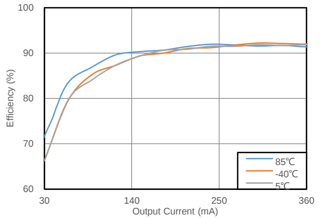
图 8.2 转换效率 vs 输出电流
