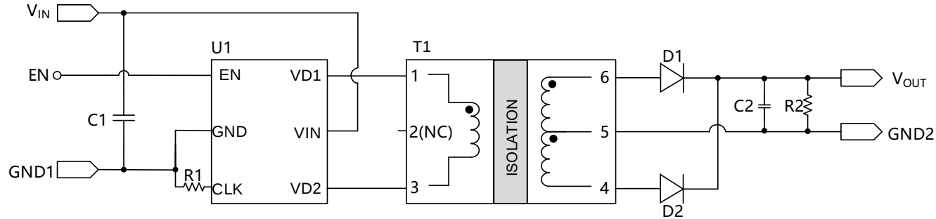
图 9.1 设计原理图
