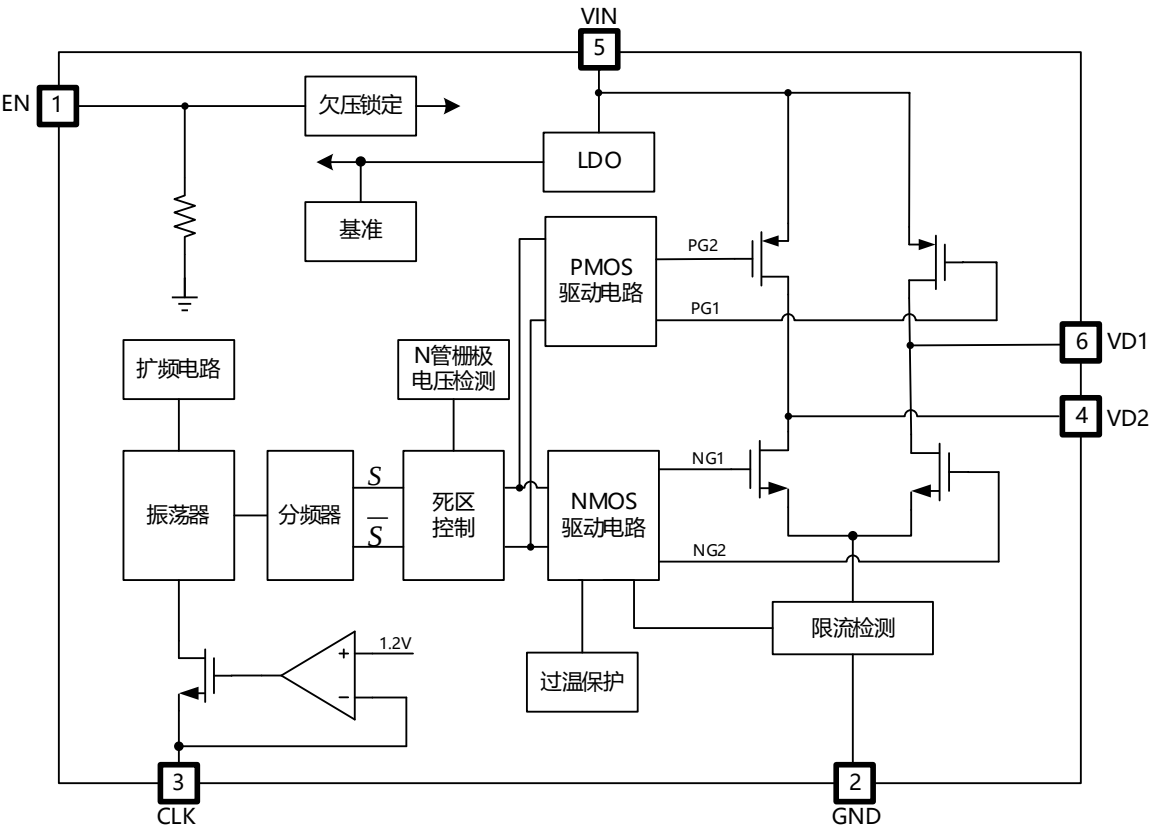
图 7.1 功能框图
