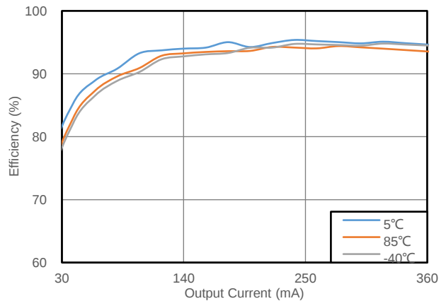
图 8.4 转换效率 vs 输出电流
