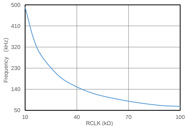
图 8.5 工作频率 vs CLK 电阻
