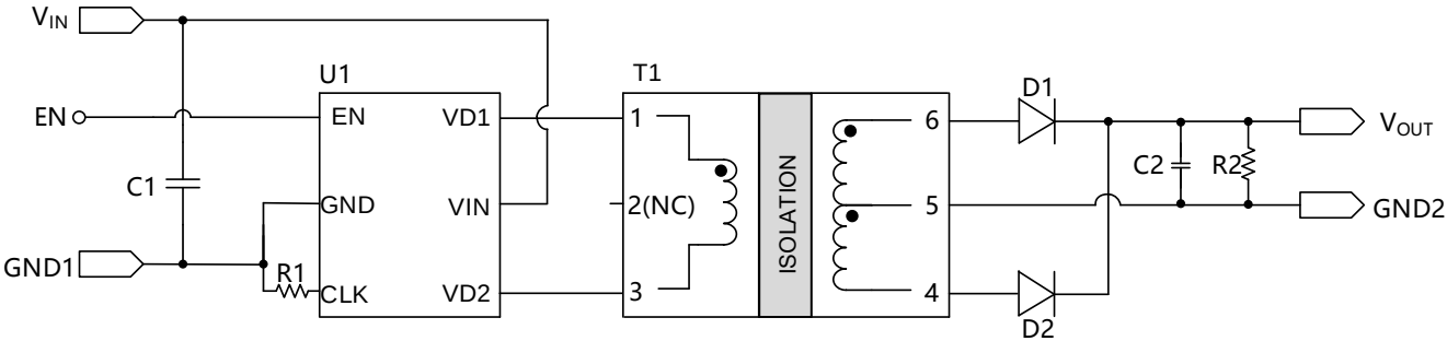
图 9.1 设计原理图
