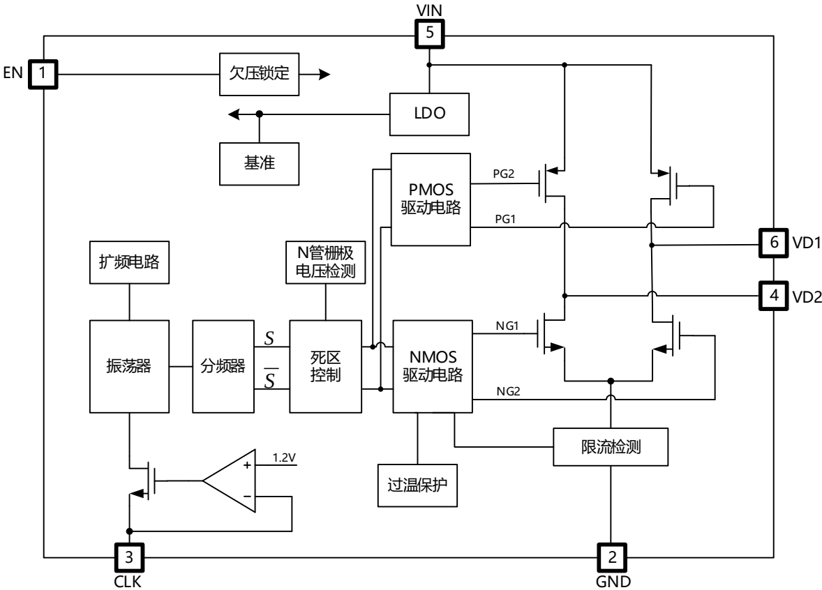
图 7.1 功能框图
