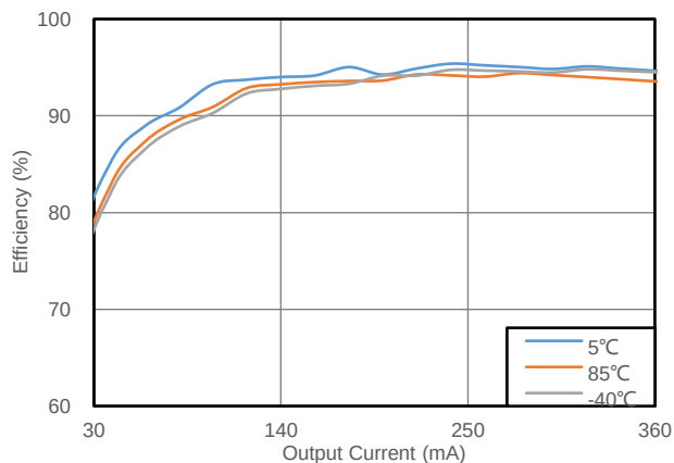
图 8.4 转换效率 vs 输出电流 (CMP6713HV+CMT78G6N, 24V to 15V, CLK=15KΩ)
