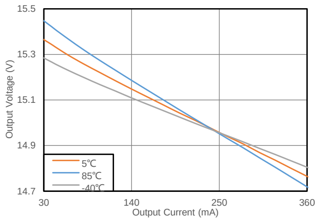
图 8.3 输出电压 vs 输出电流 (CMP6713HV+CMT78G6N, 24V to 15V, CLK=15KΩ)
