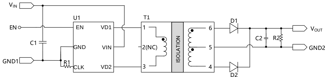
图 9.1 设计原理图
