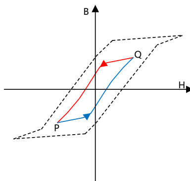
图 7.3 全桥变压器磁芯磁化曲线
