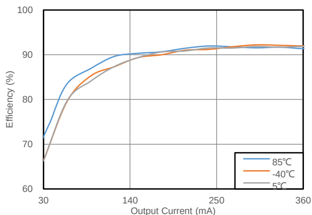
图 8.2 转换效率 vs 输出电流
