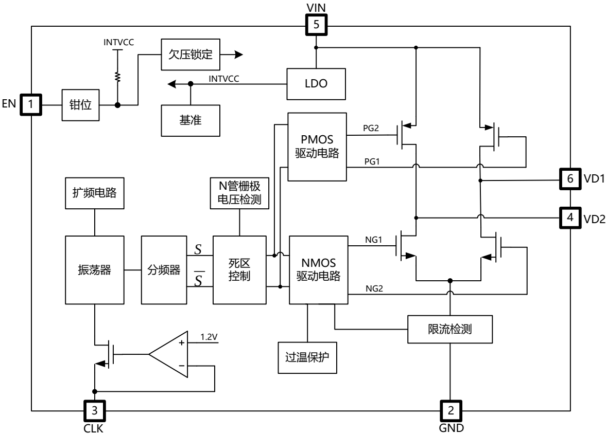
图 7.1 功能框图
