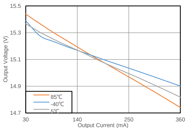
图 8.1 输出电压 vs 输出电流
