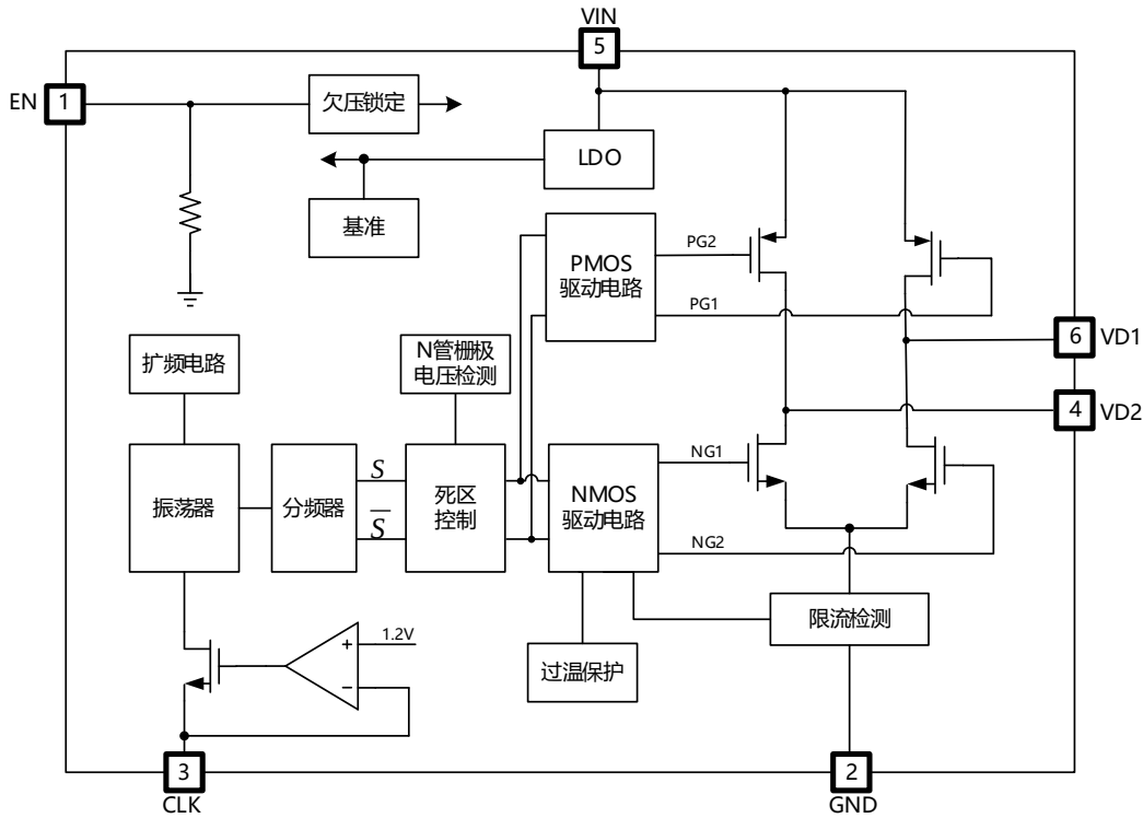
图 7.1 功能框图
