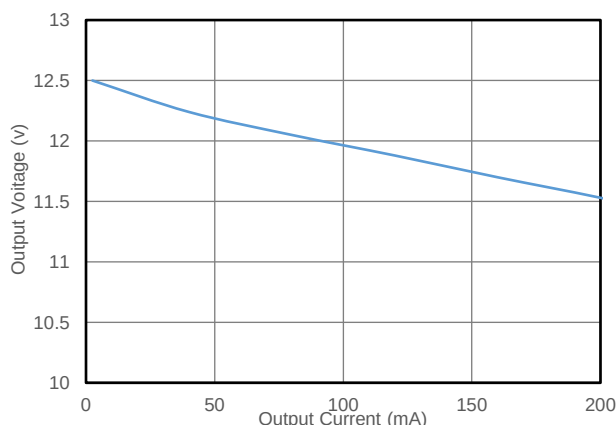
图 7.1 输出电压 vs 输出电流 (CMP6713RE+CMT78F0N, 12V to 12V, CLK=悬空)
