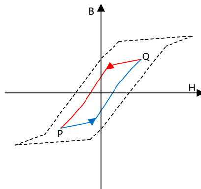
图 7.3 全桥变压器磁芯磁化曲线
