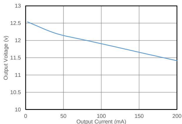
图 7.2 转换效率 vs 输出电流 (CMP6713RE+CMT78F0N, 12V to 12V, CLK=15KΩ)
