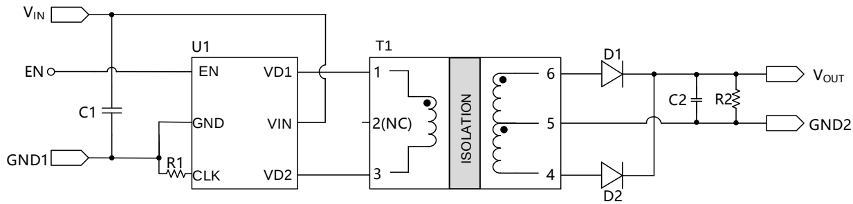
图 9.1 设计原理图
