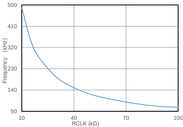
图 7.4 工作频率 vs CLK 电阻
