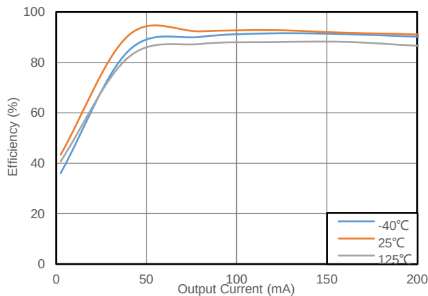
图 7.3 输出电压 vs 输出电流 (CMP6713RE+CMT78F0N, 12V to 12V, CLK=悬空)
