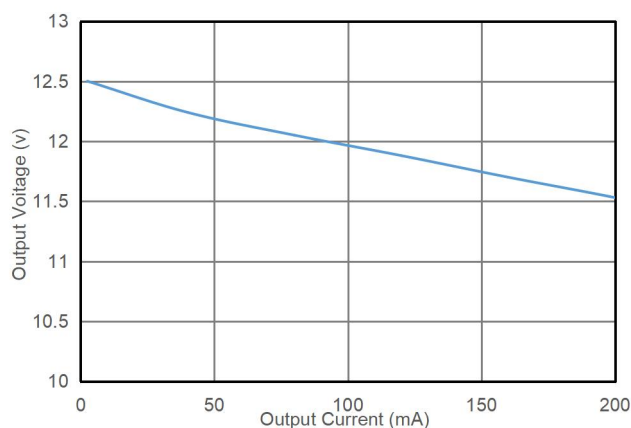
图 8.1 输出电压 vs 输出电流 (室温) (78F0N, 12V to 12V, CLK=悬空)
