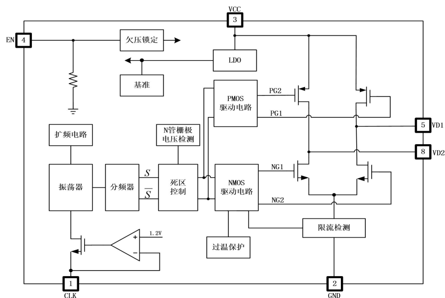
图 7.1 功能框图
