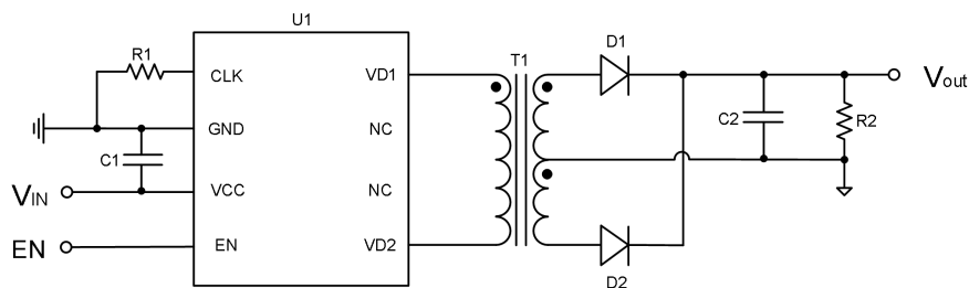
图 9.1 设计原理图
