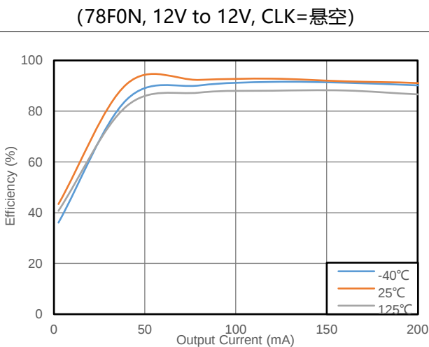
图 8.3 转换效率 vs 输出电流 (78F0N, 12V to 12V, CLK=悬空)
