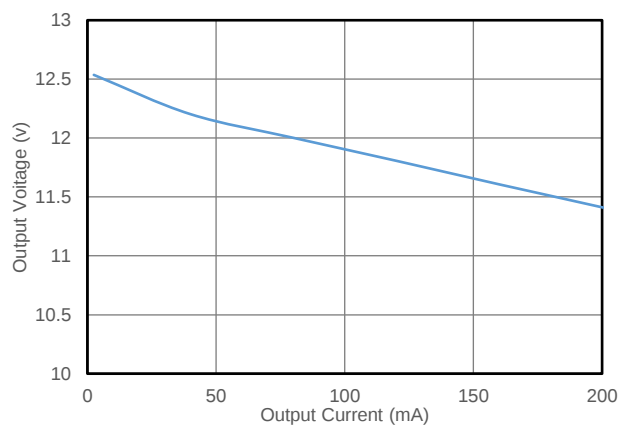
图 8.2 输出电压 vs 输出电流 (室温)
