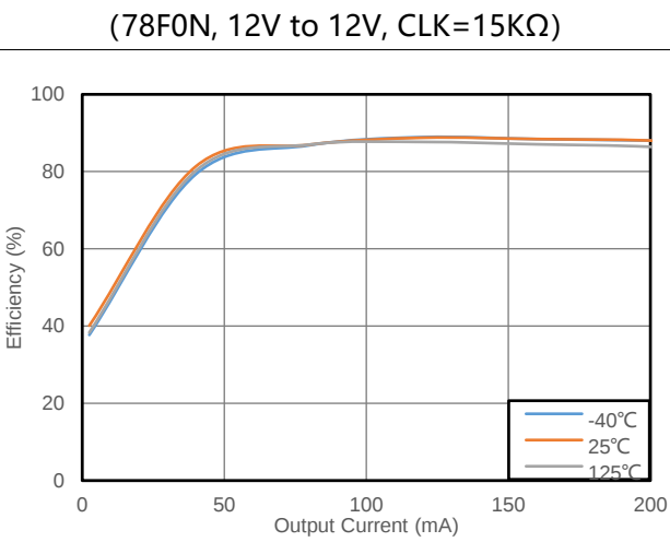
图 8.4 转换效率 vs 输出电流 (78F0N, 12V to 12V, CLK=15KΩ)
