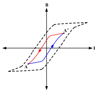
图 7.3 全桥变换器磁芯磁化曲线
