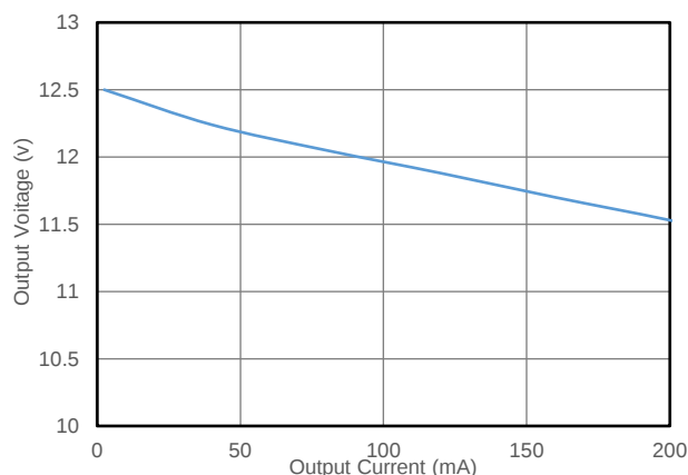
图 8.1 输出电压 vs 输出电流 (室温)
