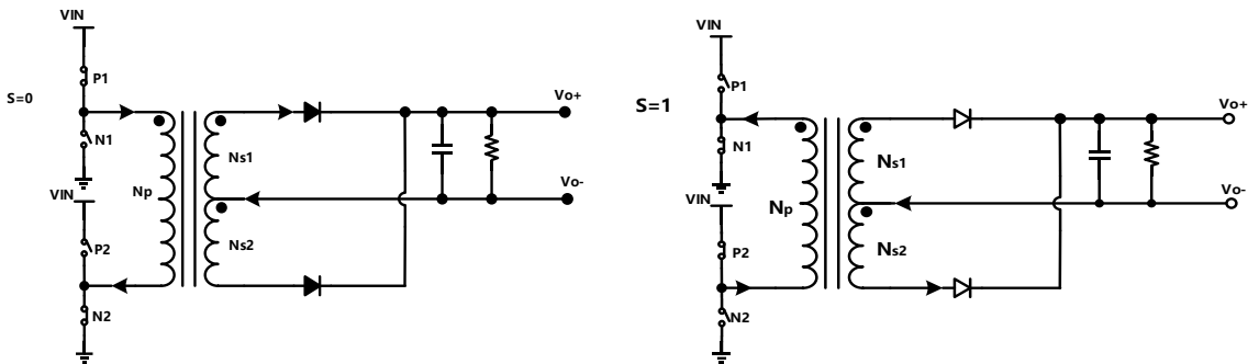
图 7.2 全桥转换器的工作过程示意图
