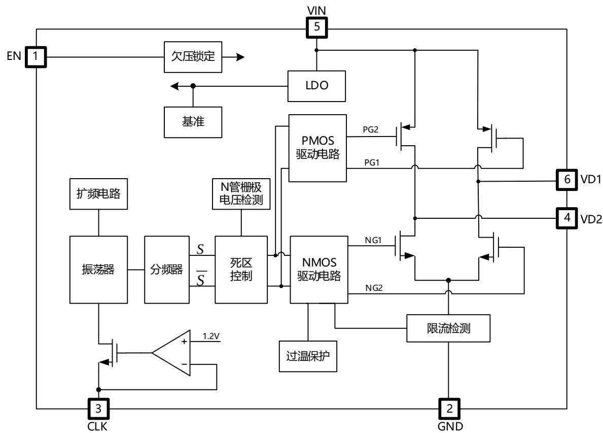
图 7.1 功能框图
