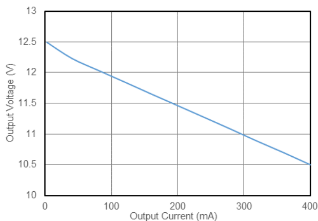
图 8.1 输出电压 vs 输出电流 (室温) CMP6793REB+CMT78F0N, 12V to 12V, CLK=悬空)
