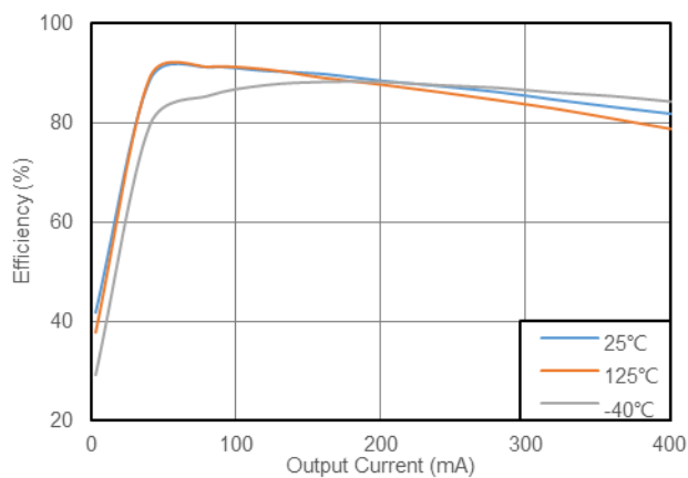
图 8.3 转换效率 vs 输出电流 (CMP6793REB+CMT78F0N,12V to12V, CLK=悬空)
