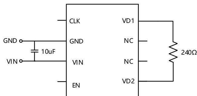
Fig. A.1 f_{sw0} \( V_{sllew} \( t_{BBM} 的测试电路
