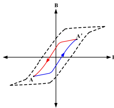
图 7.3 全桥变换器磁芯磁化曲线
