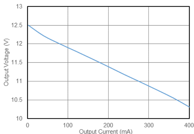
图 8.2 输出电压 vs 输出电流 (室温) (CMP6793REB+CMT78F0N, 12V to 12V, CLK=15KΩ)
