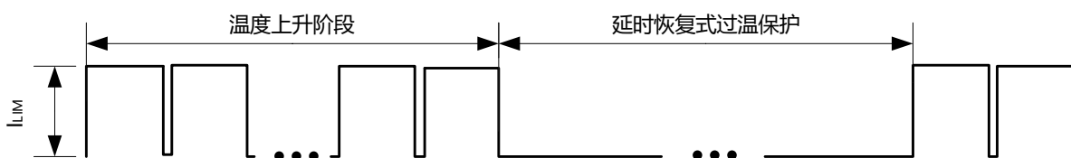
Fig. A.4 I_{LIM} 测试时序图
