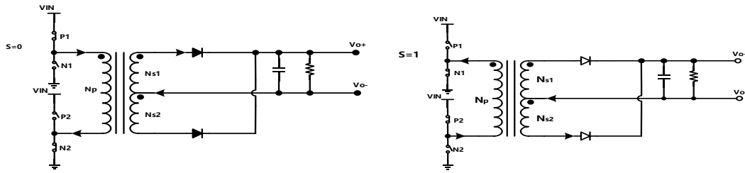
图 7.2 全桥变换器的工作过程示意图
