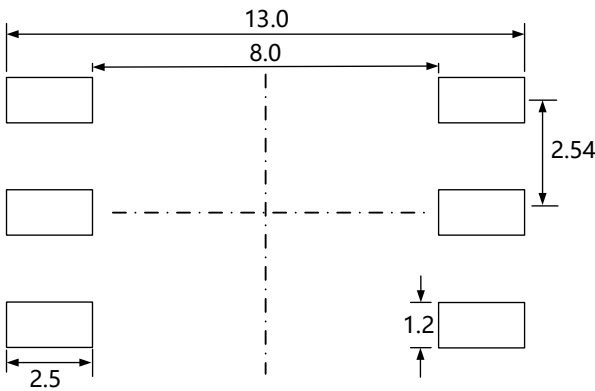
Fig. C.2 SMD-6W 建议焊盘 (所有尺寸单位为 mm)
