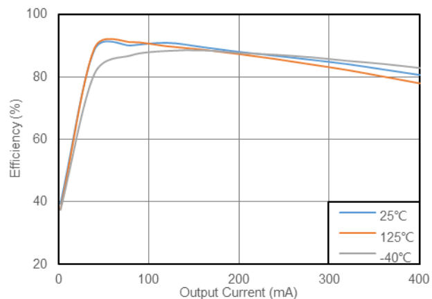
图 8.4 转换效率 vs 输出电流 (CMP6793REB+CMT78F0N,12Vto12V, CLK=15KΩ)
