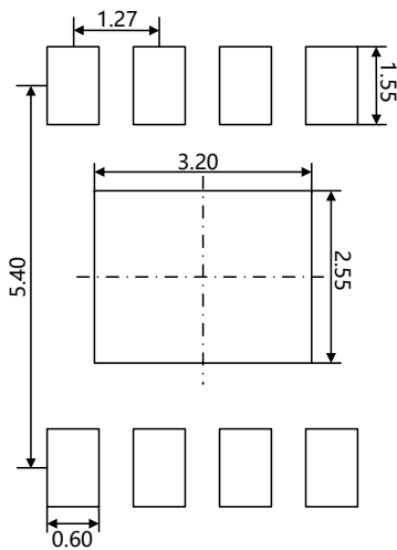
Fig. B.2 ESOP8 建议焊盘 (所有尺寸单位为 mm)
