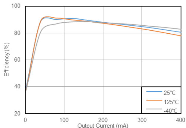
图 8.4 转换效率 vs 输出电流 (CMP6793REB+CMT78F0N,12V to12V, CLK=15KΩ)
