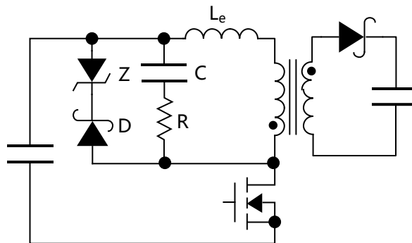
图 7.3 (RC+DC) 缓冲电路
