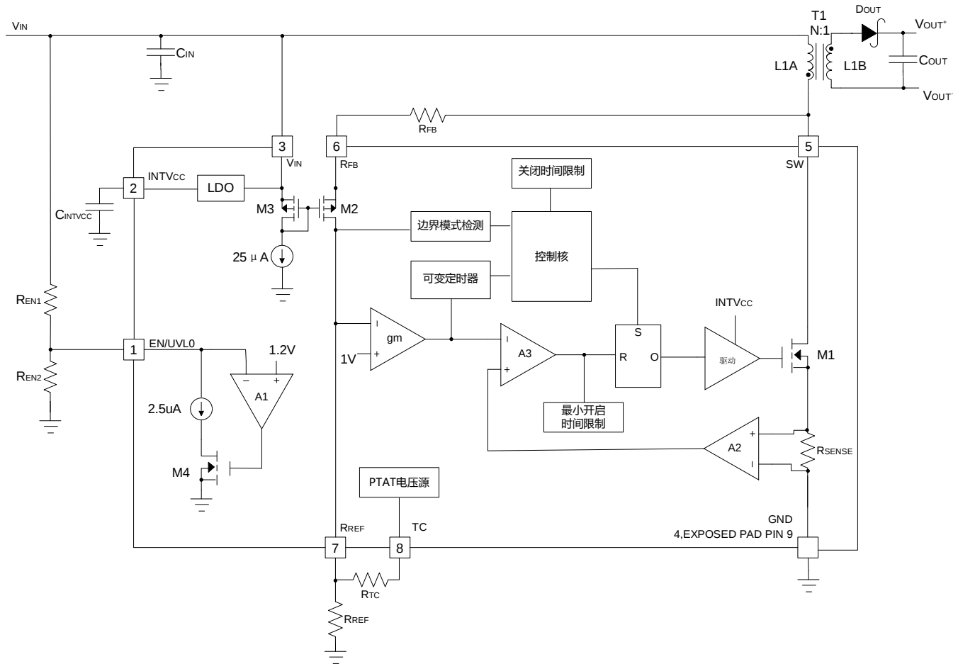
图 7.4 系统框图
