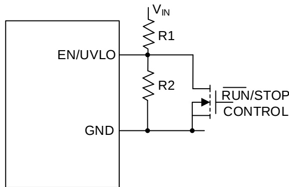
图 7.1 欠压锁定 (UVLO)
