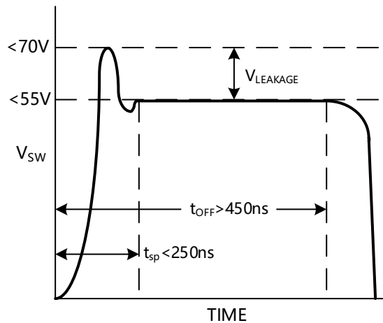
图 7.2 初级反馈波形的最大电压
