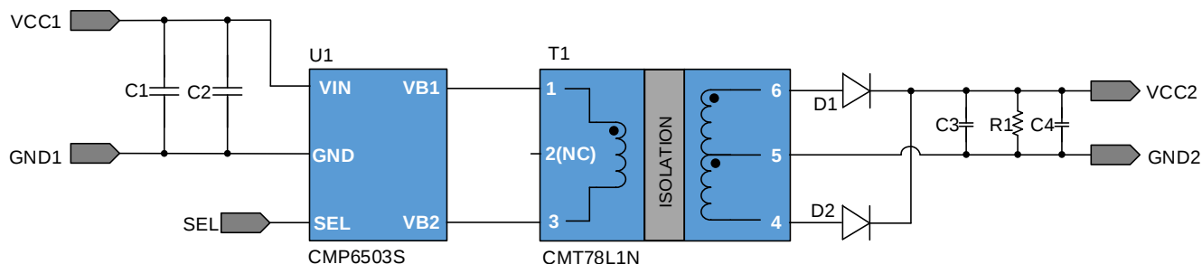
图 3.1 CMP6503S 5V 输入, 3.3V 输出 1W 方案原理图
