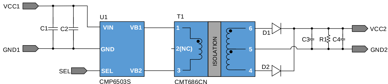
图 3.1 CMP6503S 5V 输入, 12V 输出 1W 方案原理图
