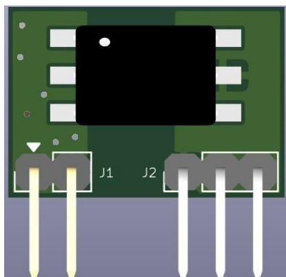
图 3.2 PCB 版图正面
