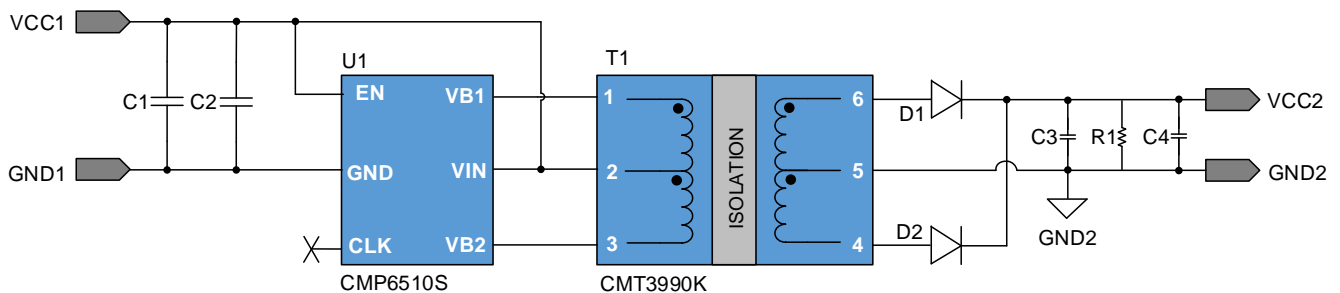
图 3.1 CMP6510S 5V 输入, 5V 输出 1W 方案原理图
