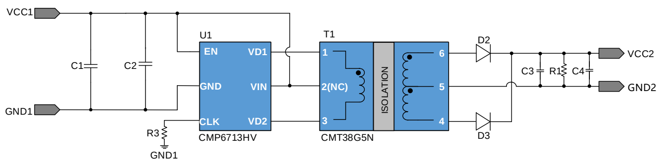
图 3.1 CMP6713HV 12V 输入, 5V 输出 1W 方案原理图
