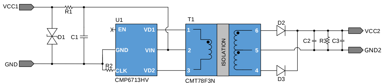
图 3.1 CMP6713HV 15V 输入, 5V 输出 2W 方案原理图
