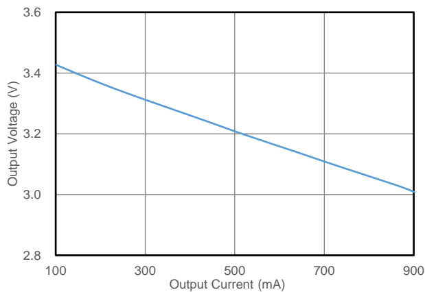
图 5.3 输出电压 vs 输出电流 (CLK 连接 15 kΩ)
