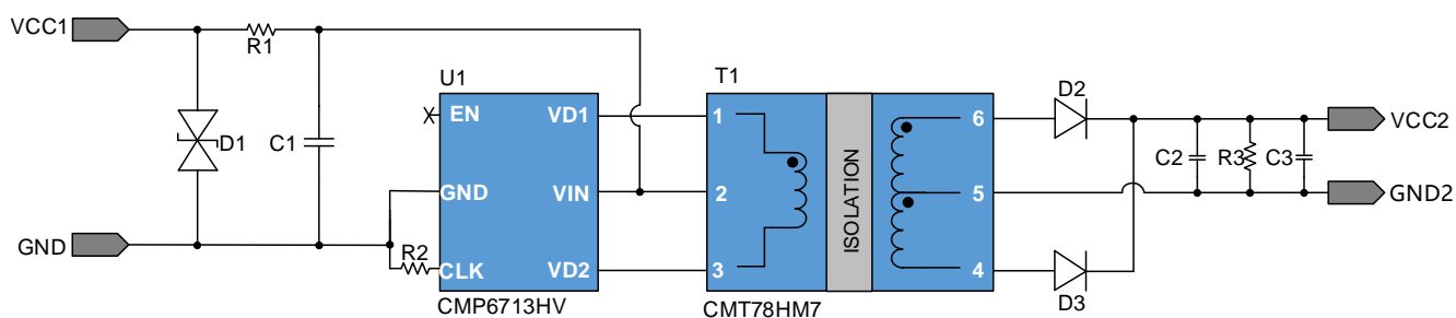
图 3.1 CMP6713HV 24V 输入, 3.3V 输出 3W 方案原理图
