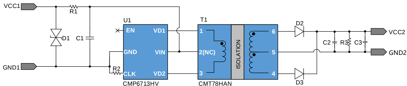
图 3.1 CMP6713HV 24V 输入, 5V 输出 3W 方案原理图
