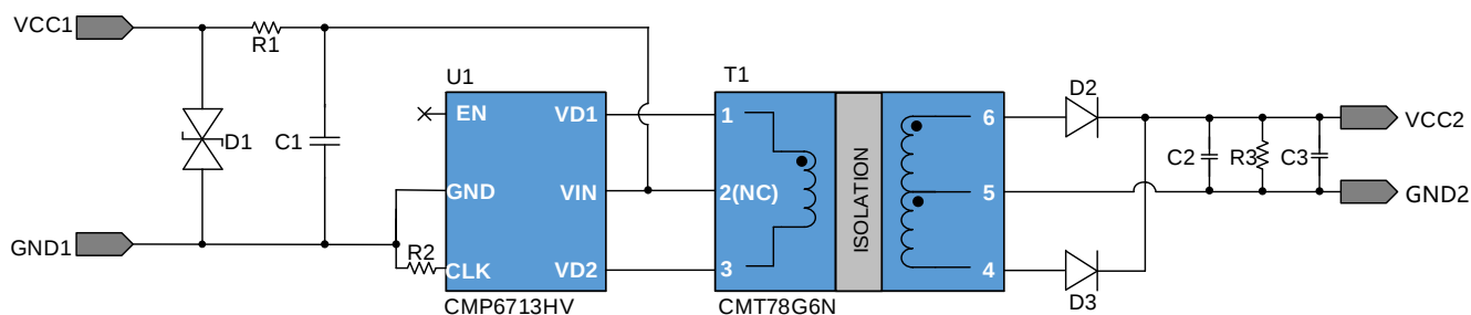
图 3.1 CMP6713HV 24V 输入, 15V 输出 6W 方案原理图
