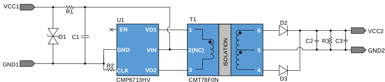
图 3.1 CMP6713HV 24V 输入, 24V 输出 6W 方案原理图
