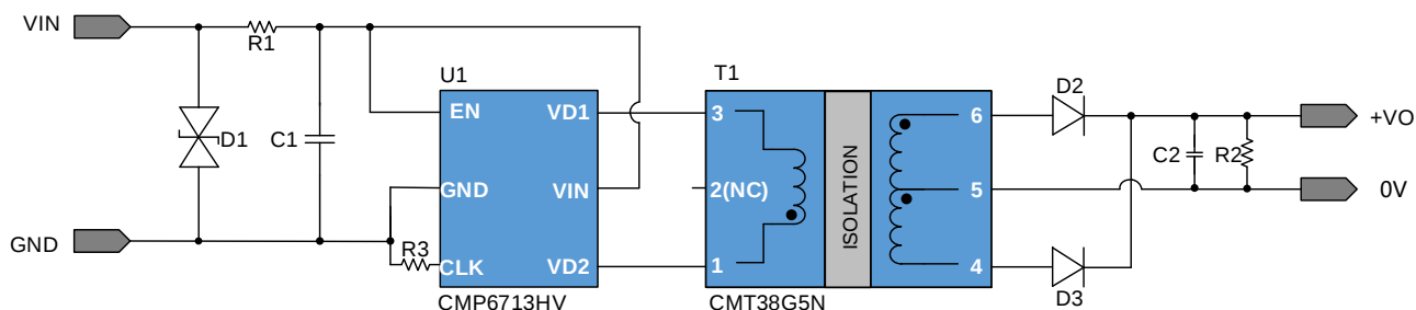
图 3.1 CMP6713HV 12V 输入, 5V 输出 1W 方案原理图
