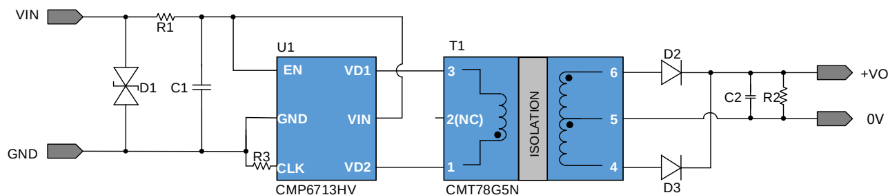
图 3.1 CMP6713HV 12V 输入, 5V 输出 2W 方案原理图
