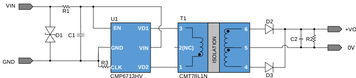
图 3.1 CMP6713HV 12V 输入, 9V 输出 2W 方案原理图
