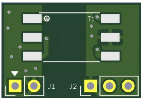
图 3.4 PCB 版图正面
