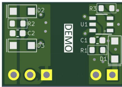
图 3.5 PCB 版图背面
