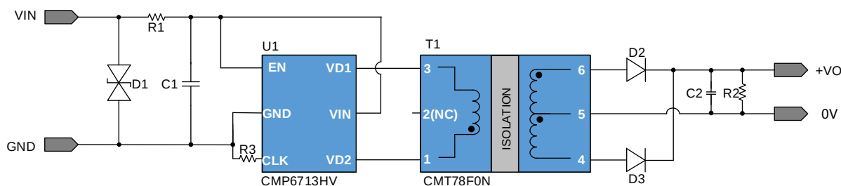
图 3.1 CMP6713HV 12V 输入, 12V 输出 2W 方案原理图
