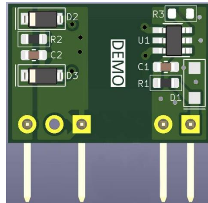
图 3.3 PCB 版图背面
